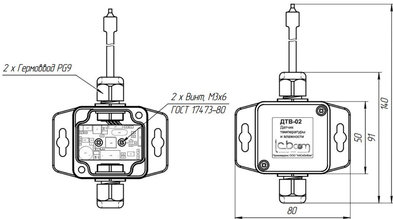
Рисунок 2 – Схема и габаритные размеры ДТВ-02
