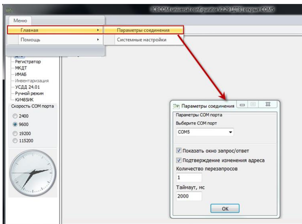
Рисунок 5 – Главное окно конфигуратора. Настройка соединения
